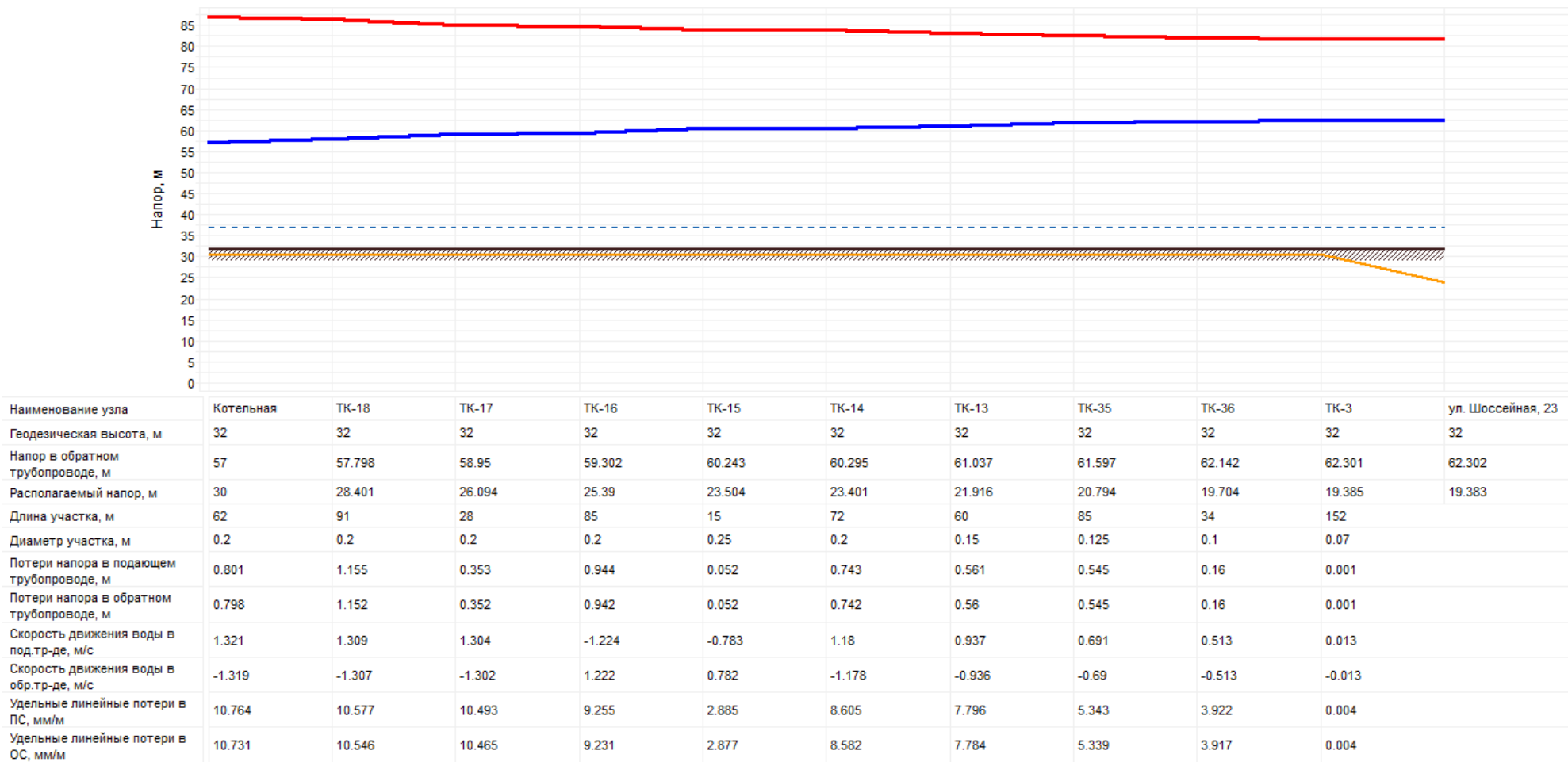
Рисунок 6.2 Пьезометрический график от котельной до здания МБОУ "Петровская СОШ"
